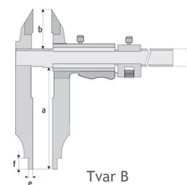
Monoblok Nonius 1/20 = 0,05 mm + 1/128"
